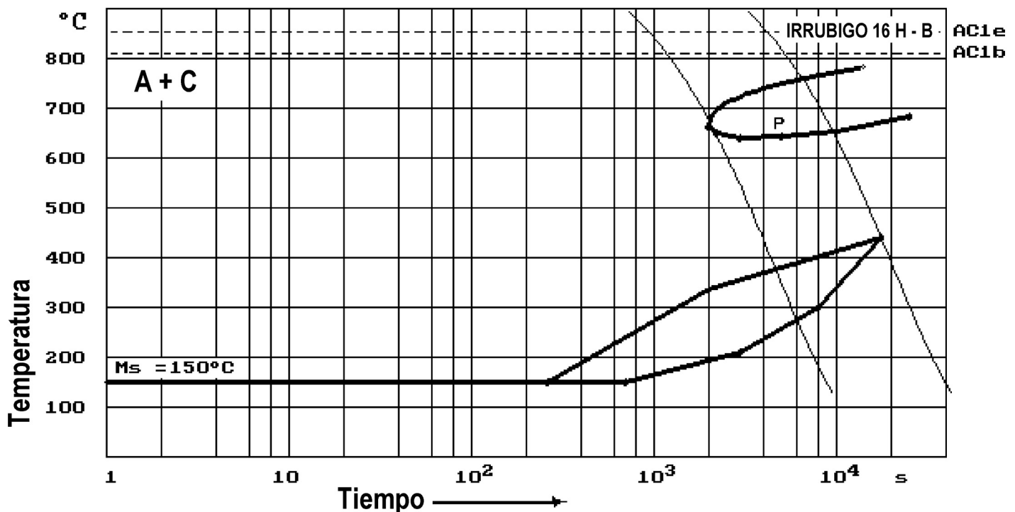
Figura 2.- Gráfico CCT.
